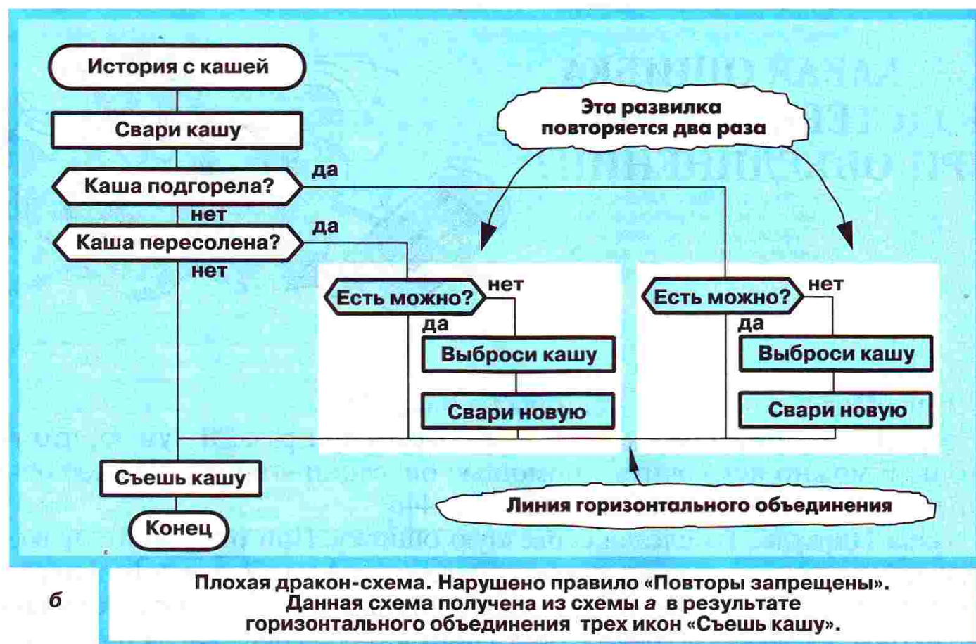
Рис. 43. Последовательное применение операций «Горизонтальное объединение» и «Вертикальное объединение» позволяет устранить ненужные повторы и превратить очень плохую (неэргономичную) дракон-схему в хорошую (эргономичную)
