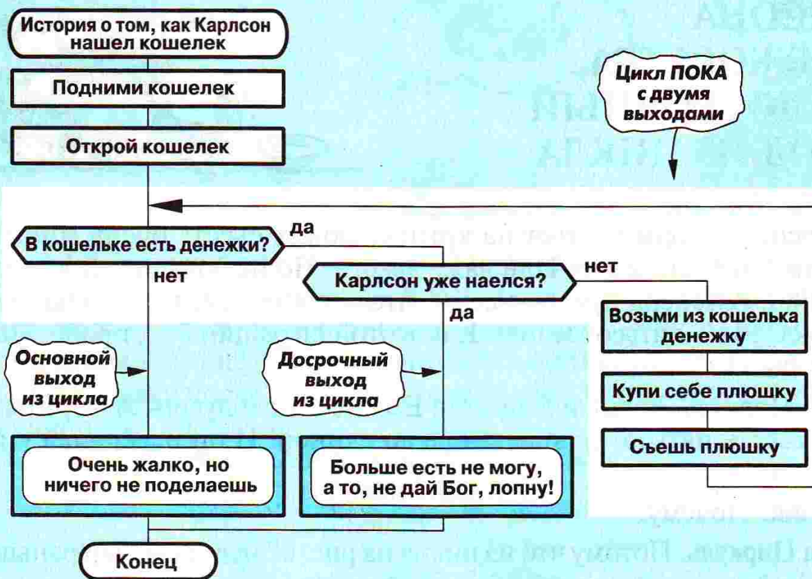
Рис. 72. Досрочный выход из цикла происходит потому, что Карлсон больше не хочет есть. Сравни с рис. 67
