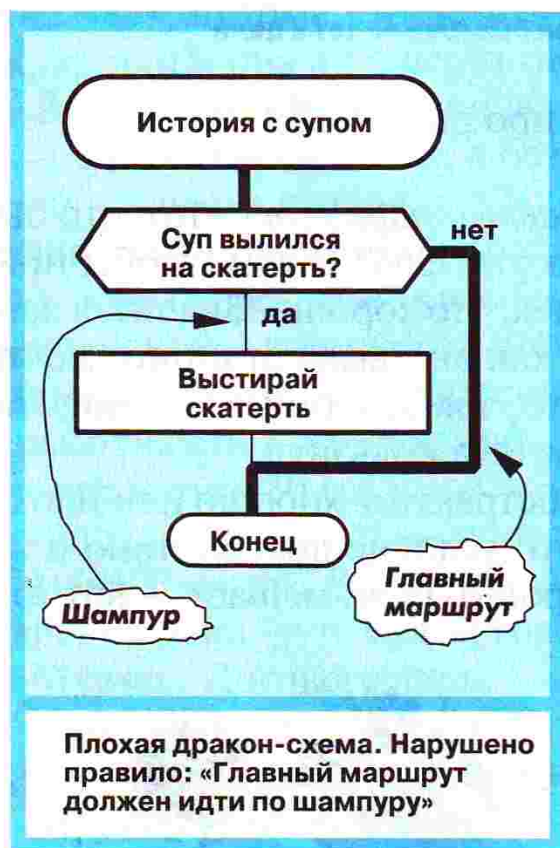
Рис. 37. Как пустить главный маршрут по шампуру? Поменяйте местами плечи у развилки
