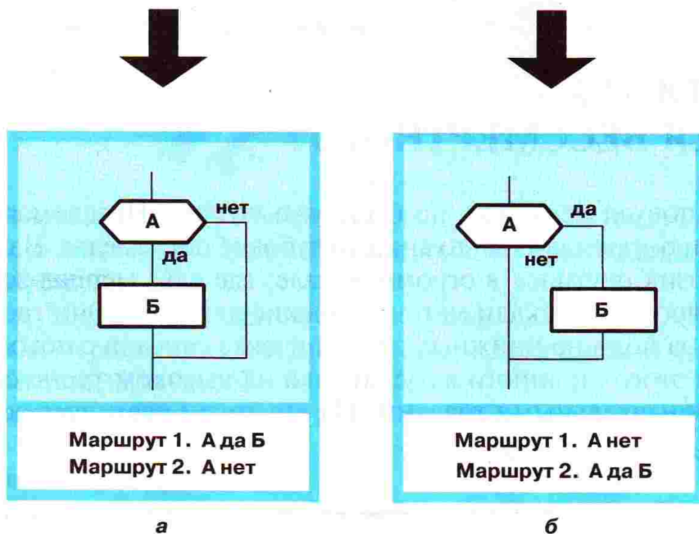
Рис. 35. Буквенные дракон-схемы, полученные из смысловых дракон-схем на рис. 34
