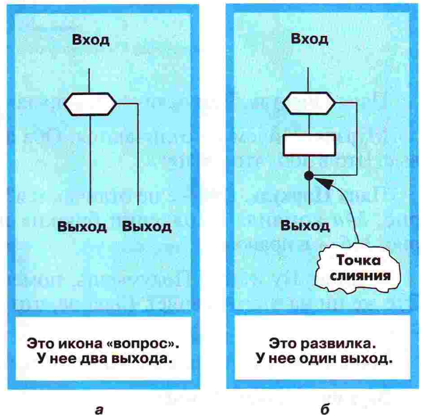
Рис. 33. Чем отличается развилка от иконы «Вопрос»?
