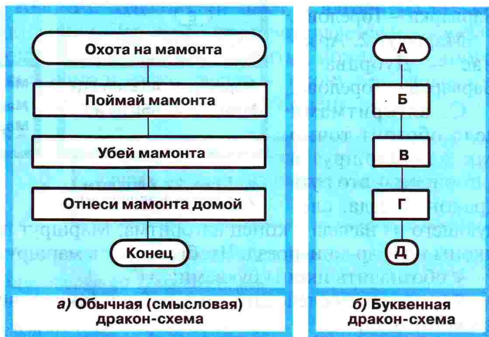
Рис. 22. Как преобразовать обычную дракон-схему в буквенную?
