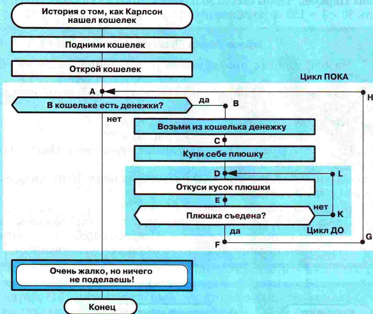
Рис. 78. Цикл в цикле. Внутри цикла ПОКА находится цикл ДО. Сравни с рис. 67
