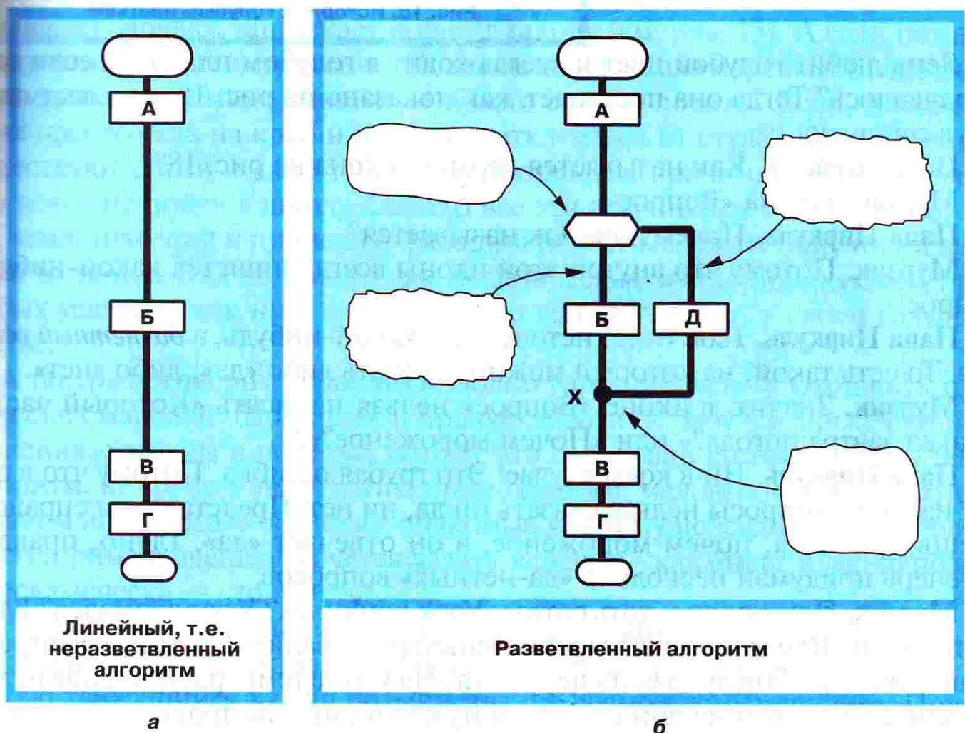
Рис. 17. Линейный и разветвленный алгоритмы
