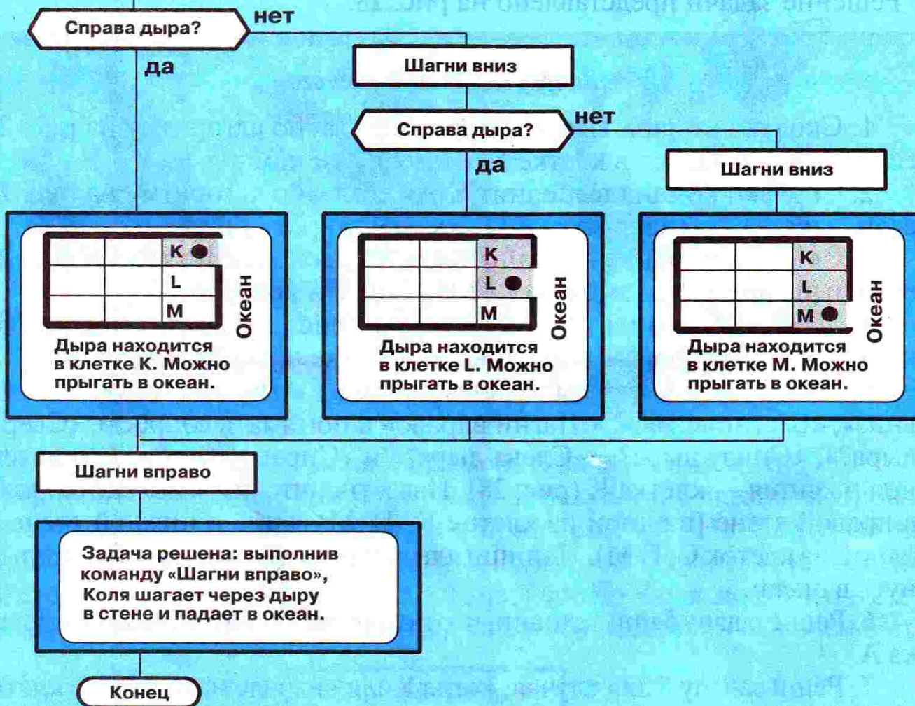
Рис. 28. Алгоритм «Робот Коля решил утопиться»
